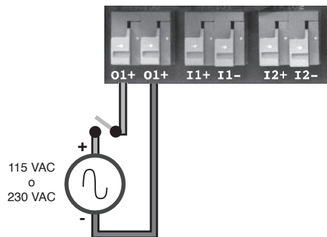
Figura 18 - Ejemplo de relé de Salida con suministro externo
